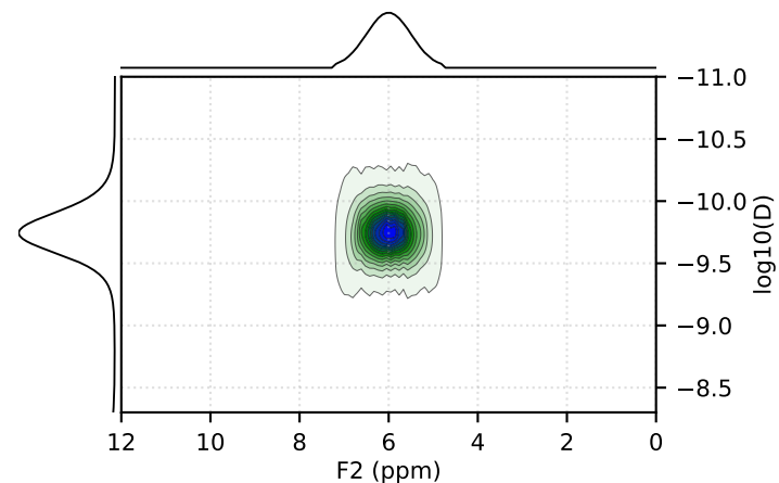
S5 (Xu) - True
