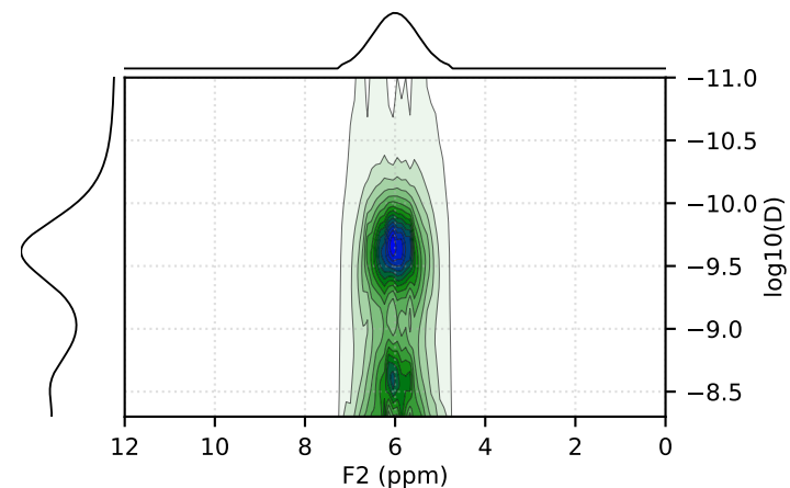
S3 (Sparse) - True
