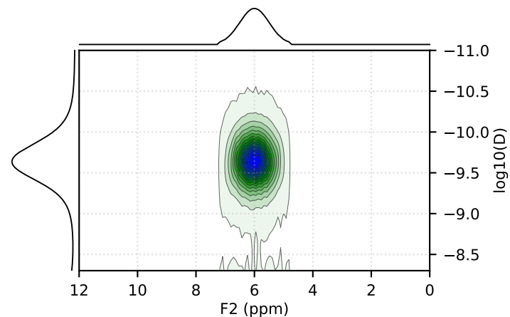
S4 (Gauss) - True
